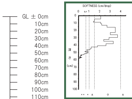
土壌貫入計 (長谷川式) S値グラフ (cm/drop)
