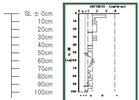
土壌貫入計 (長谷川式) S値グラフ (cm/drop)
