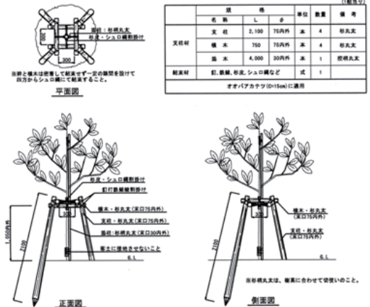
図 -3.3 支柱の規格
