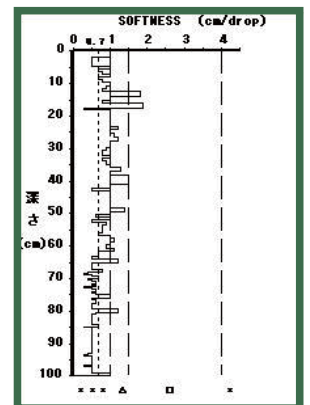
土壌貫入計 (長谷川式) S値グラフ (cm/drop)
