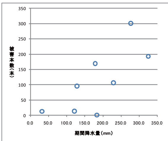
図-1.23 期間降水量と被害本数の関係
