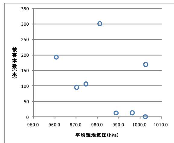
図-1.24 平均現地気圧と被害本数の関係
